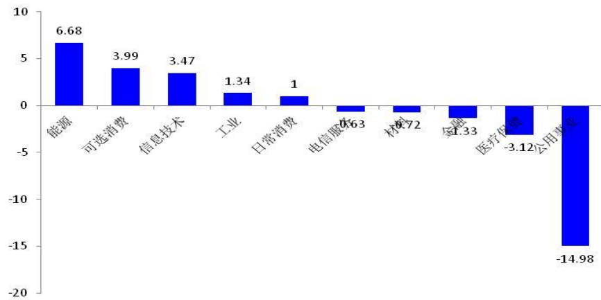
图 11 能源板块表现最佳 板块之间涨幅差异大
