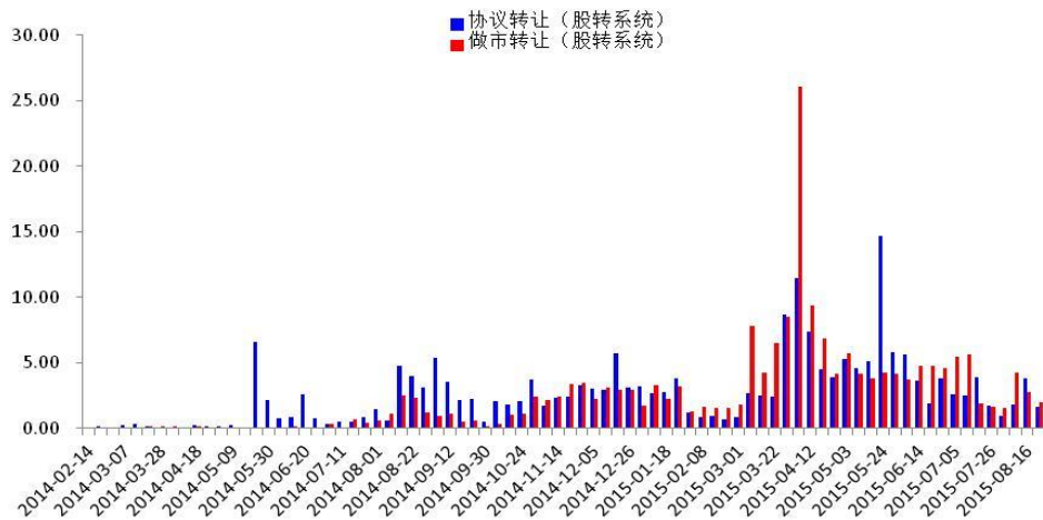
图 5 成交金额环比前一周大幅下降 协议转让尤甚
