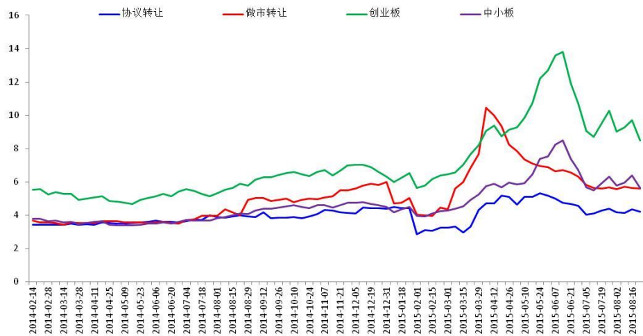
图 9 协议转让企业和做市转让企业 PB 分别为 4.21 倍和 5.59 倍
