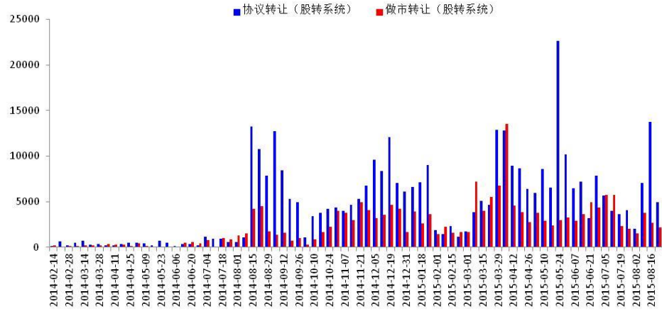
图 4 转让成交股票总量环比前一周大幅下降 协议转让尤甚
