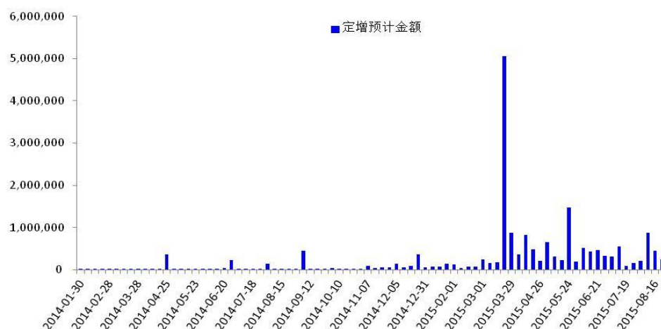
图 13 预计定增募集资金大幅下降 下降幅度为 46.71%
