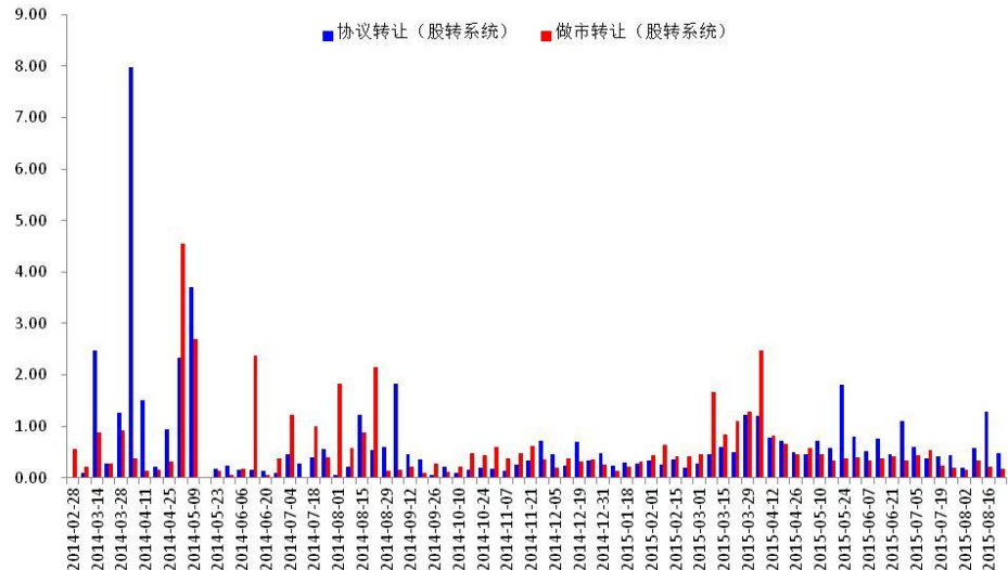
图 6 换手频率窄幅波动
